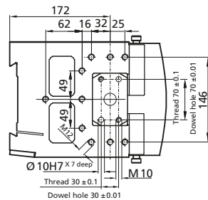
Press Type 368
