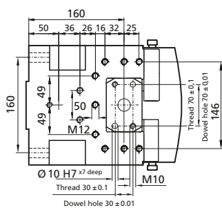
Press Type 364
