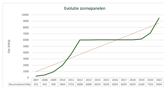
Grafiek: evolutie van het geïnstalleerd vermogen zonnepanelen van Ecopower sinds 2007
