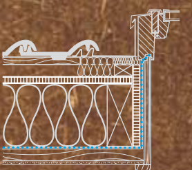
Het kan nochtans anders: detail van een wind-, water- en luchtdichte uitvoering met de isolerende Celit 4D onderdakplaat.
