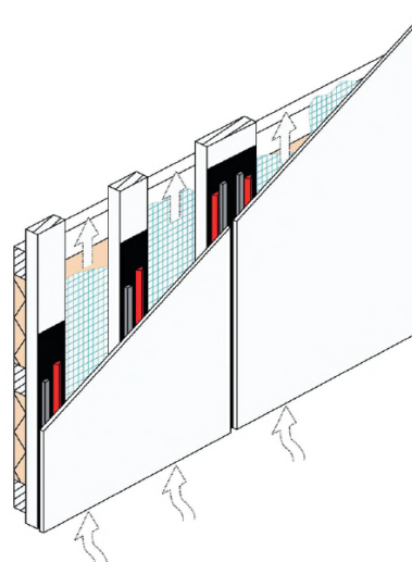
Detail ventilatie
