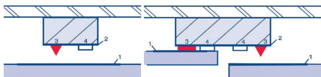
Detail gevelpanelen verlijmen
