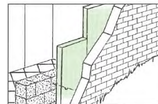
Sponning
