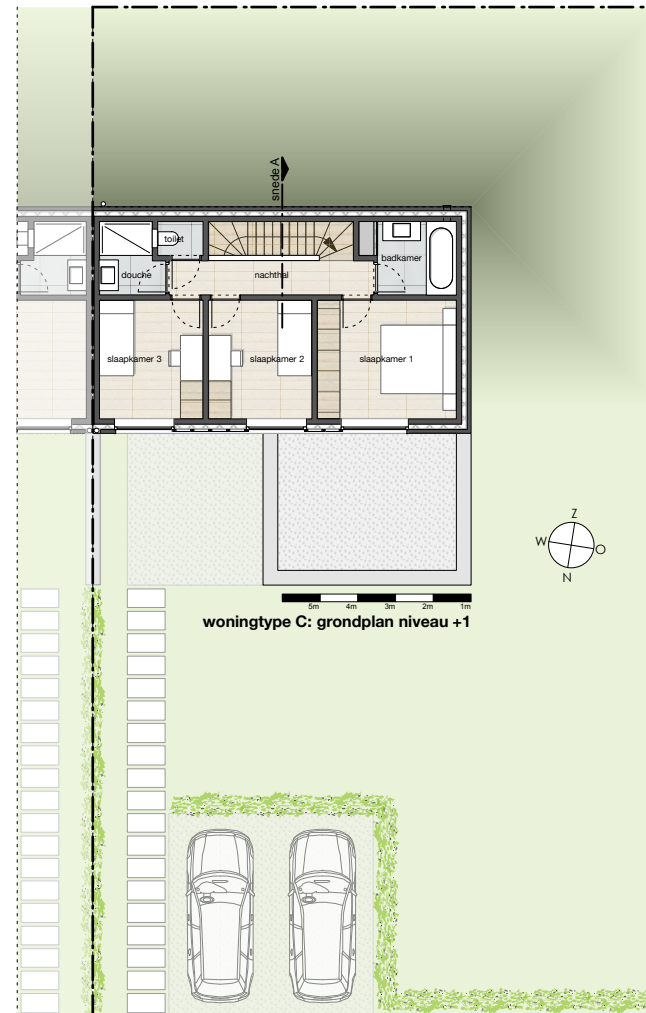
woningtype C: grondplan niveau +1
