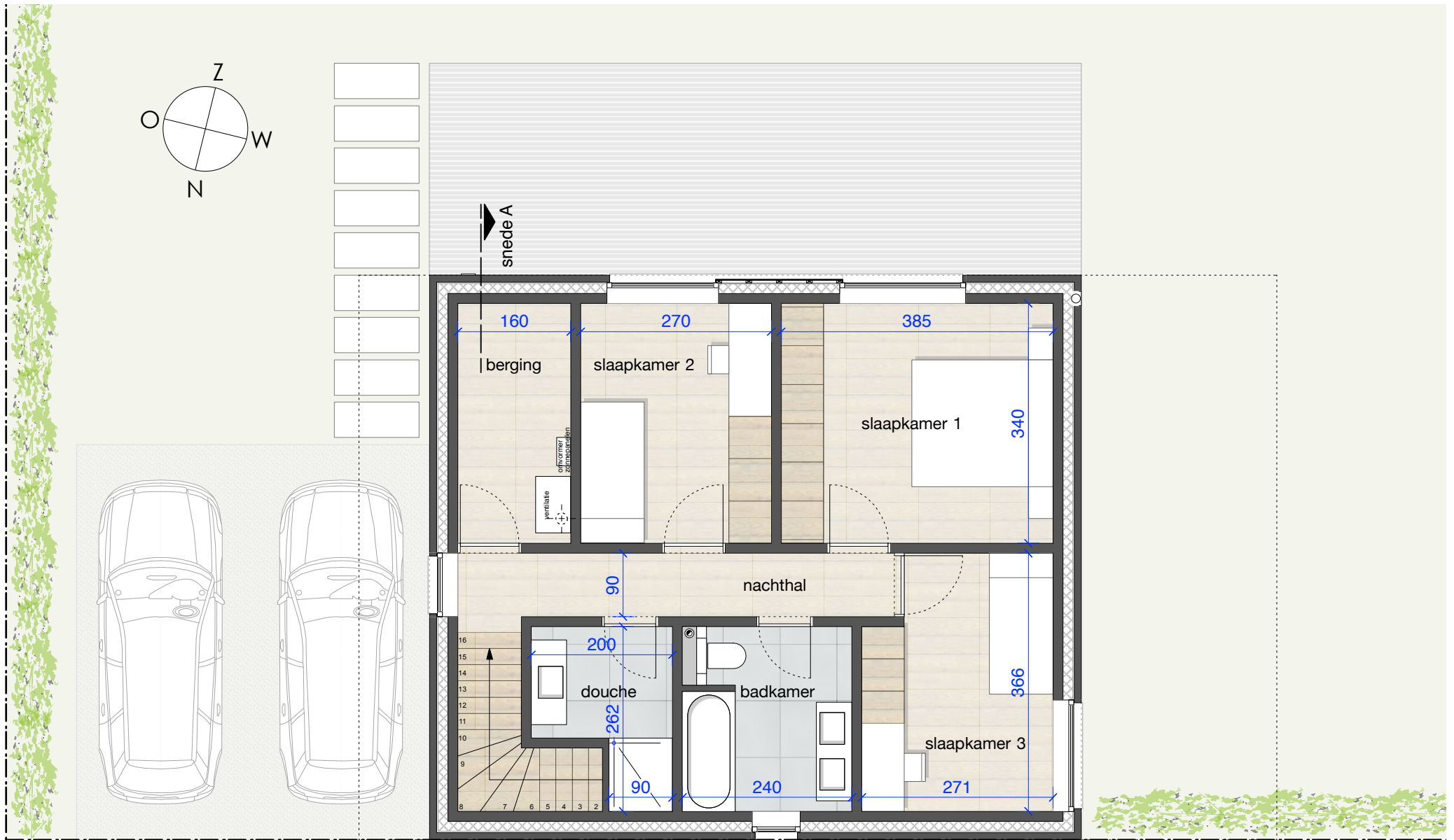
woningtype D: gronplan niveau +1, variante 1
